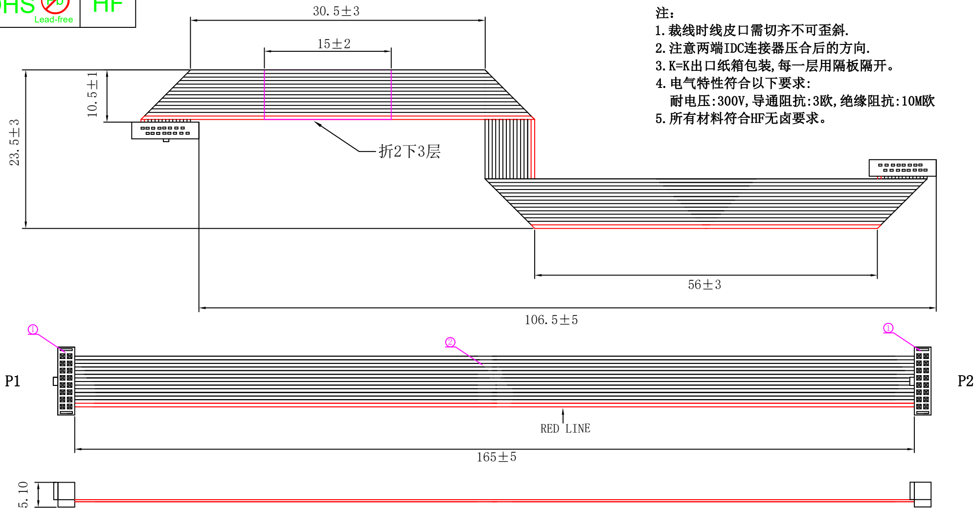
接点图:
